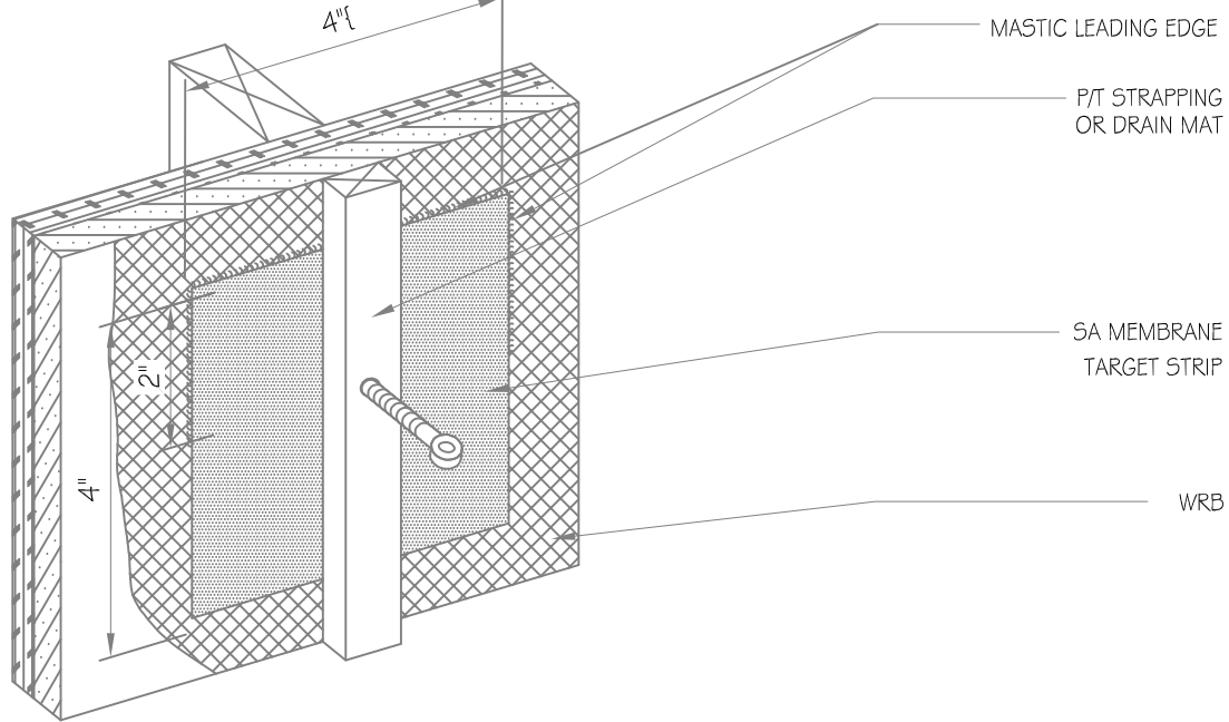
12A SCAFFOLD ANCHOR BE-2.3 SCALE: NTS
